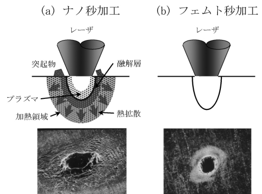
Fig. 1 レーザパルス幅による加工の違い
