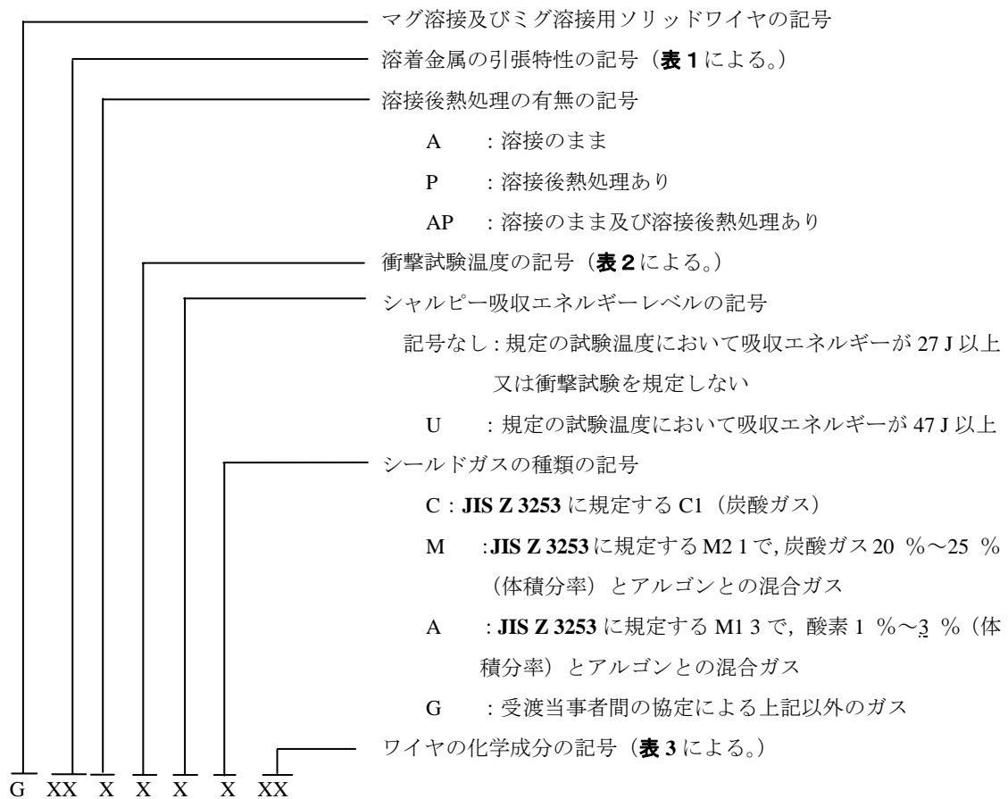
図 1 ISO に基づいたワイヤの種類の記号の付け方
