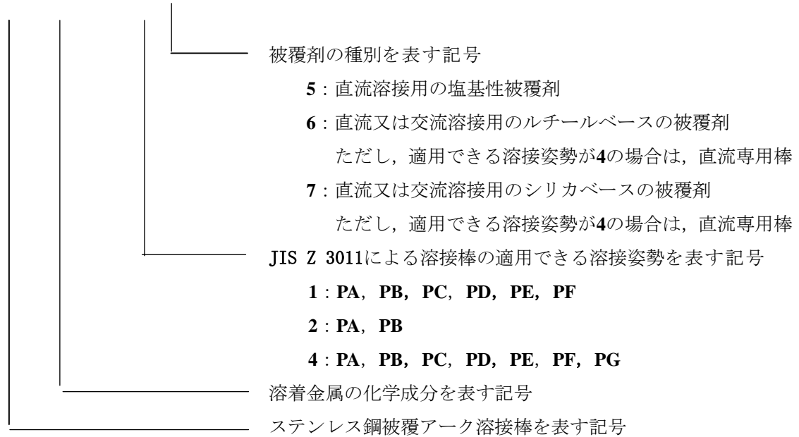
図1—ステンレス鋼被覆アーク溶接棒の種類の記事の付け方
