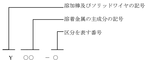
図 2-a 現行 JIS Z 3334 : 1999 溶加棒及びソリッドワイヤの種類の記号の付け方
