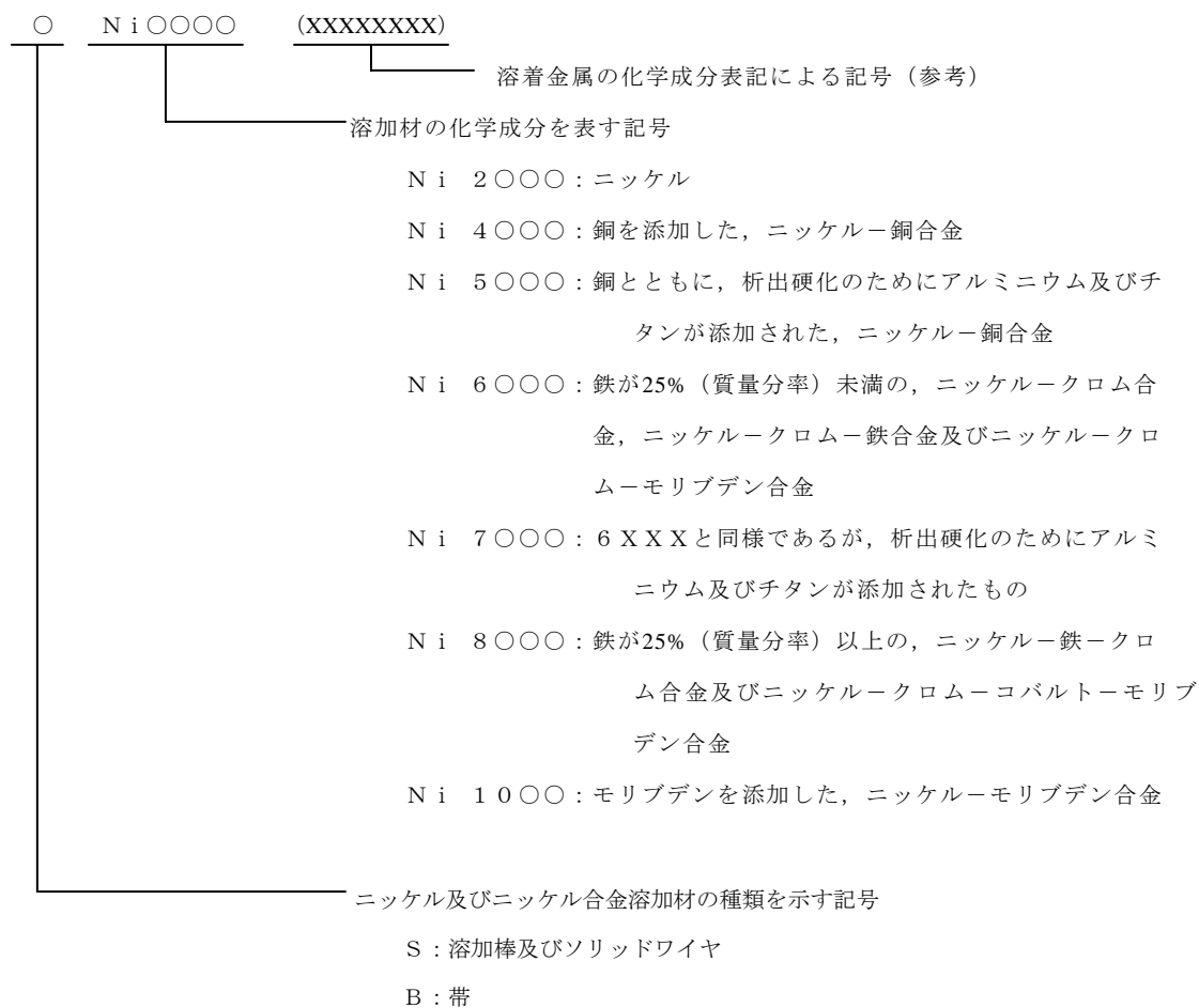
図 2-b JIS Z 3334 改正案の溶加棒, ソリッドワイヤ及び帯の種類の記号の付け方
